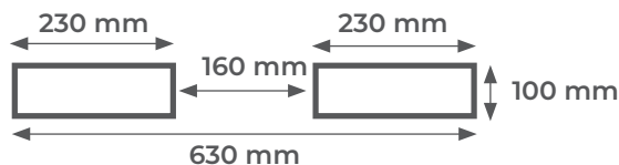
Dimensions intérieures des fourreaux BAS200 à BAS300
